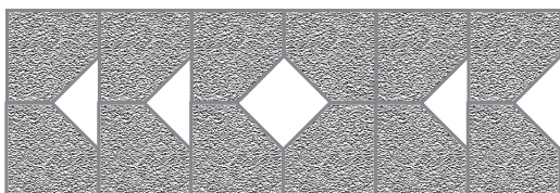
Formação 4 - Bandeirinha Mista Escala 1:20
